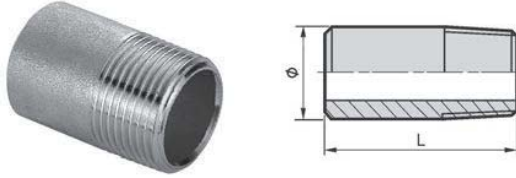
型式:R-7C
