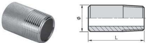
型式:R-7F
