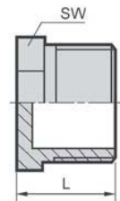
型式:R-8 単位:mm
