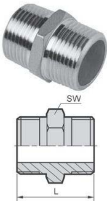
型式:R-72(NPT/PT) 単位:mm
