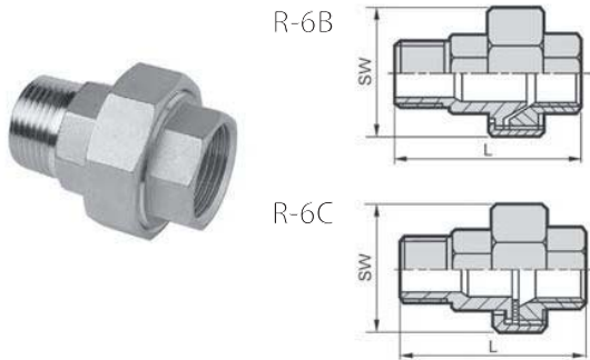
型式:R-6B 単位:mm
