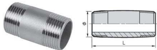
型式:R-7B 単位:mm
