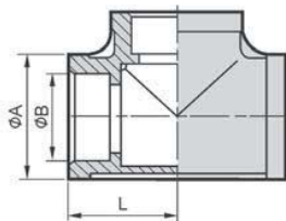
型式:R-2B 単位:mm
