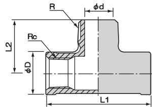
型式:R-2F 単位:mm
