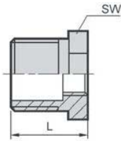
型式:R-9 単位:mm
