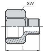
型式:R-9A 単位:mm
