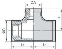
型式:R-2A 単位:mm
