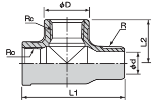
型式:R-2E 単位:mm
